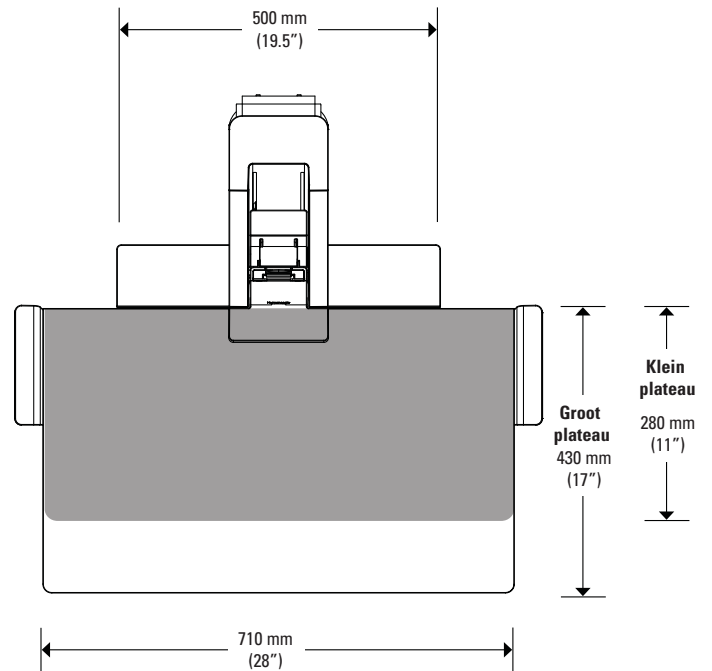
Zijaanzicht
