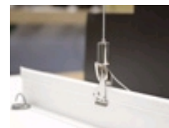
Ophanging met spiraal anker en hoofdprofiel
