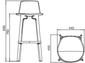
Taburete altura alta Stool high back
