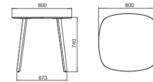
Mesa encimera 80x80 Table top 80x80
