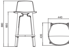
Taburete altura media Stool medium back
